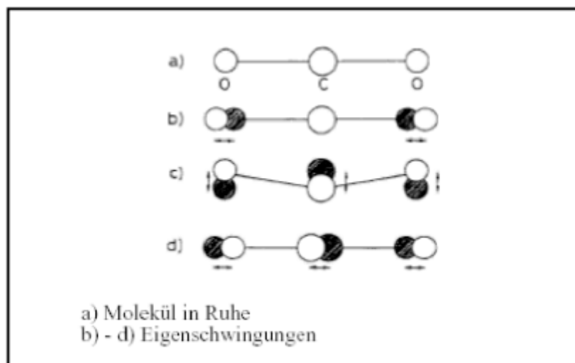
Bild 4: Schwingungsarten ("Moden") des 3-atomigen CO 2 -Moleküls
