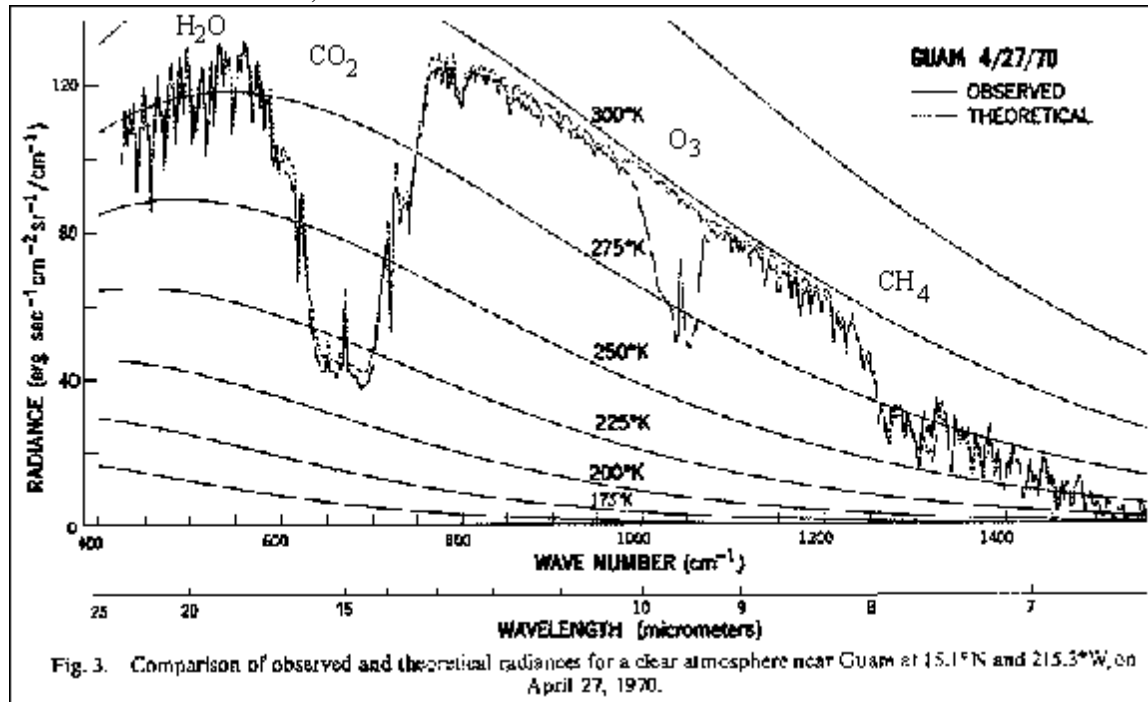
Bild 5: Spektrum der Erdatmosphäre, aufgenommen im Infrarotbereich von einem Erdsatelliten aus, bei klarer Luft am 27.4.1970 über der Pazifikinsel Guam
